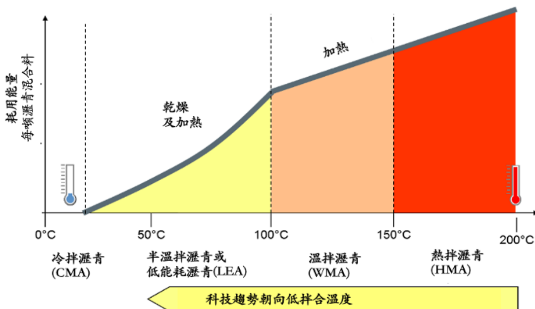
三種加熱拌合瀝青的拌合溫度界限及能耗示意圖
