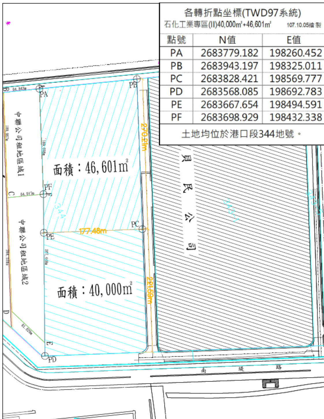
臺中港石化工業專區貝民南側土地位置平面圖
